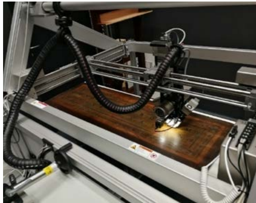
Ruckers virginaal in de CT scan, TU Delft. MA-XRF van de klep van Ruckers virginaal in het Ateliergebouw, Rijksmuseum
